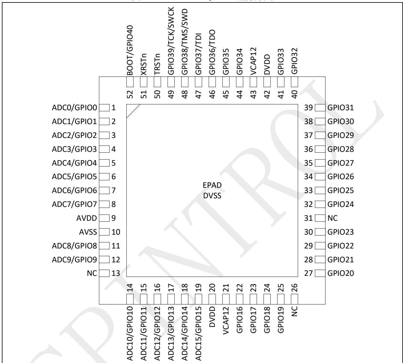
图 3-5: SPC1168 QFN52 引脚排列
