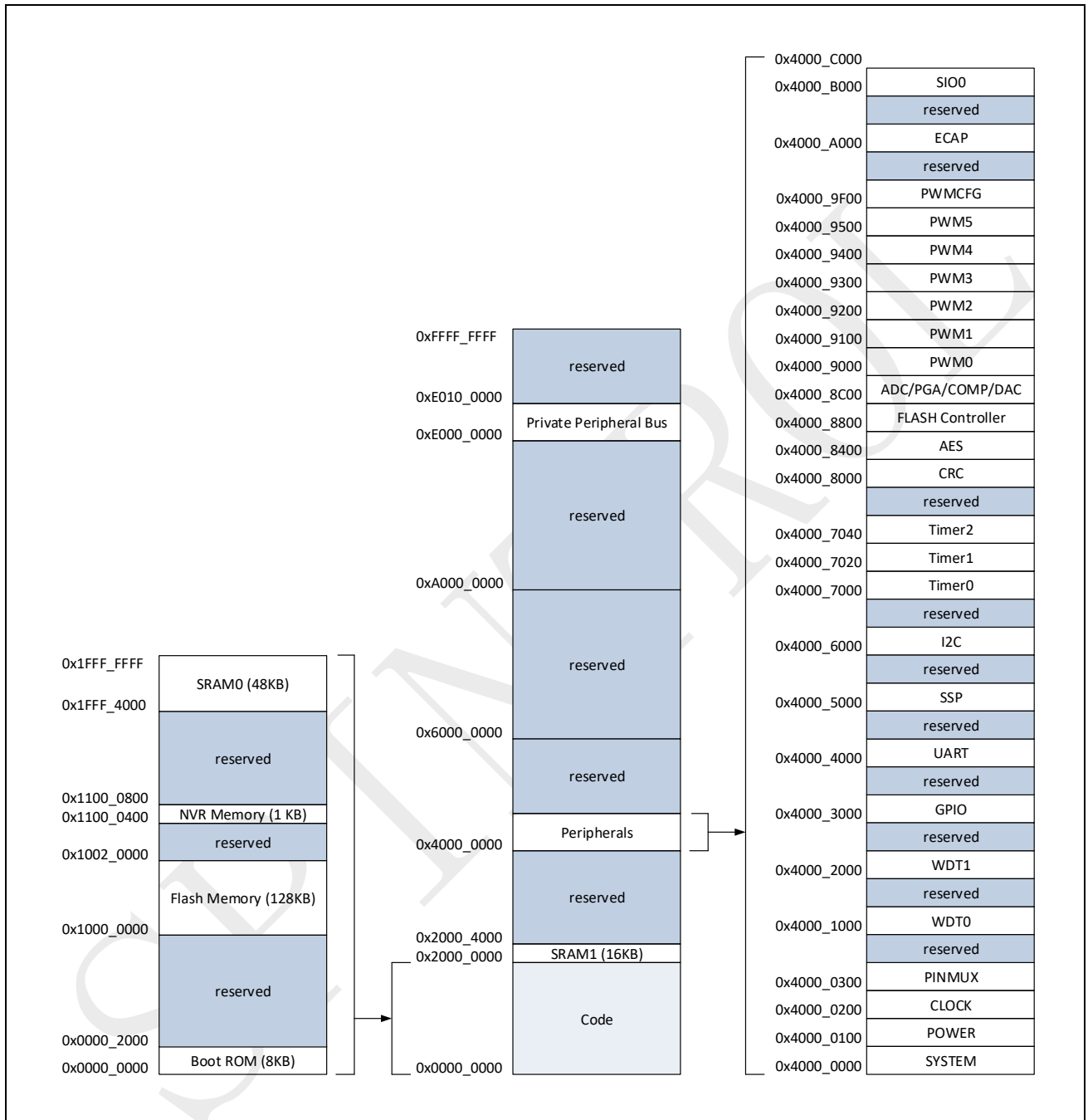
图 4-1: 存储器映射
