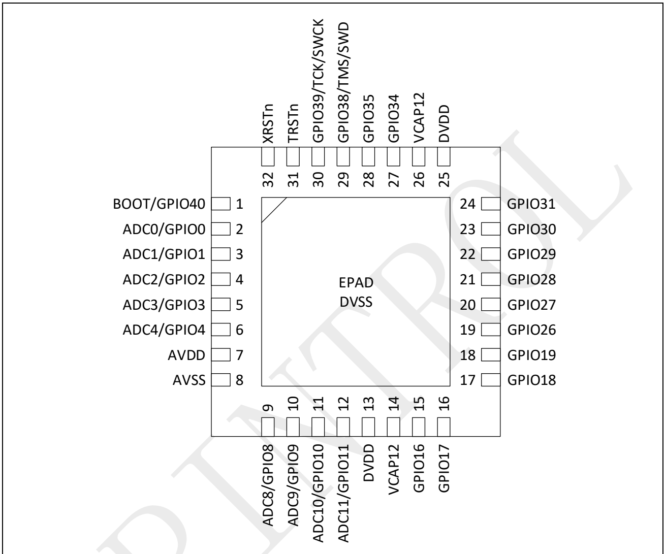
图 3-4: SPC1168 QFN32 引脚排列
