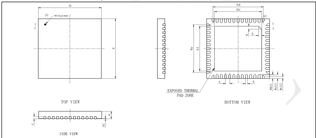
图 6-9: QFN52-52 脚, 6 x 6 mm 方形扁平无引脚封装
