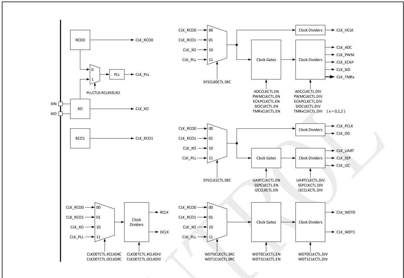
图 1-2: 时钟树
