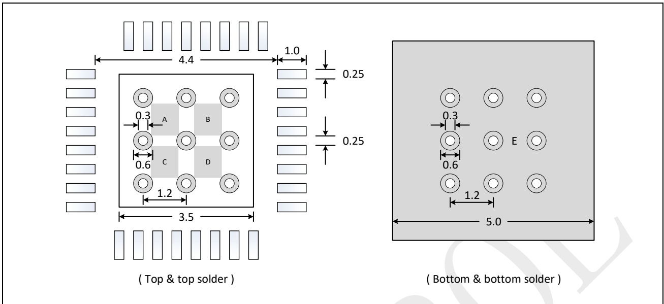
图 6-8: QFN32-32 脚, 5 x 5 mm 方形扁平无引脚封装推荐尺寸
